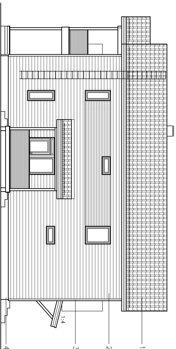
JULKISIVU ITÄÄN
